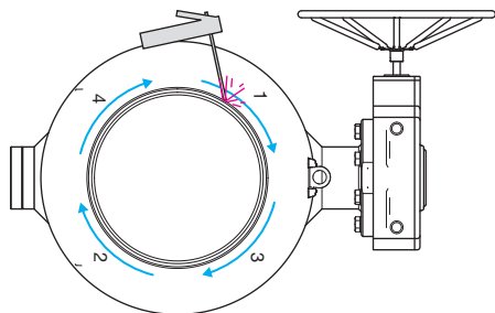
Рис. 4. Выполнение сварных швов
